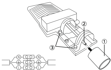
Рис. 1. Монтаж светильника
